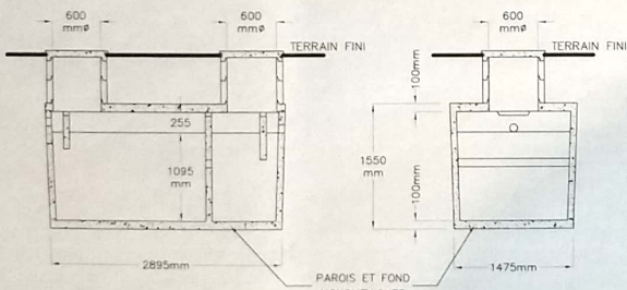
FOSSE SEPTIQUE MODELE FSM-5000 DE MEI
