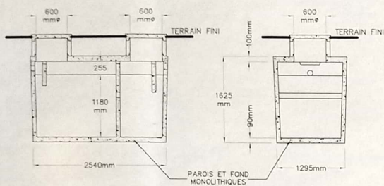
FOSSE SEPTIQUE MODELE FSM-4000 DE MEI
