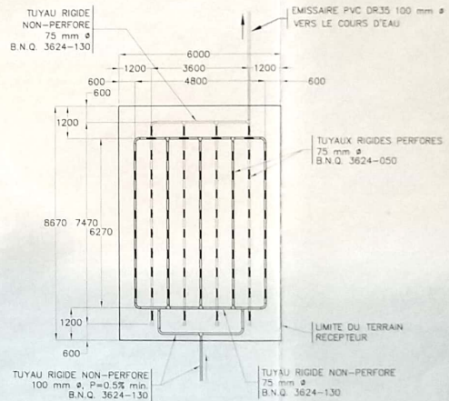
PLAN AGRANDI DU FILTRE A SABLE CLASSIQUE
